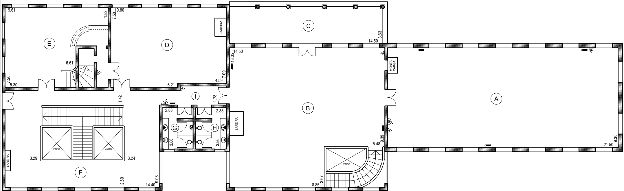
PLANTA BAIXA PAVto. SUPERIOR
